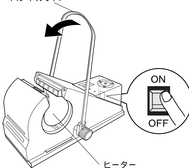
ハンドルレバー
