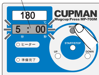
プレス時間表示
